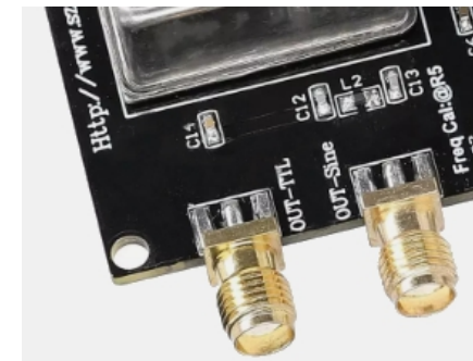
OCXO-en har både TTL og Sinus output.
